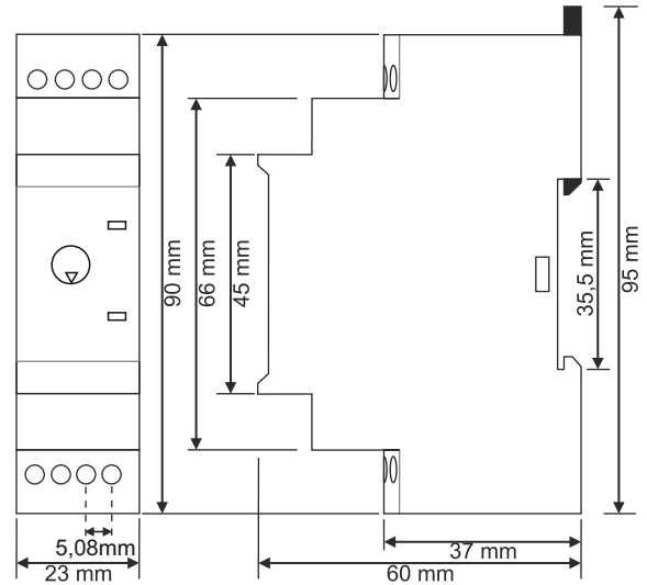
Şekil 3: Panel boyutları
