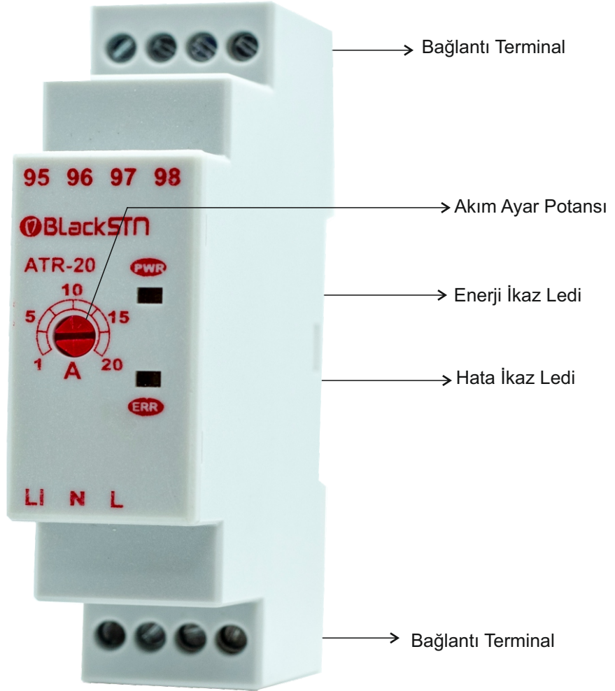
Şekil 1: Analog Termik Koruma Dış Görünüm
