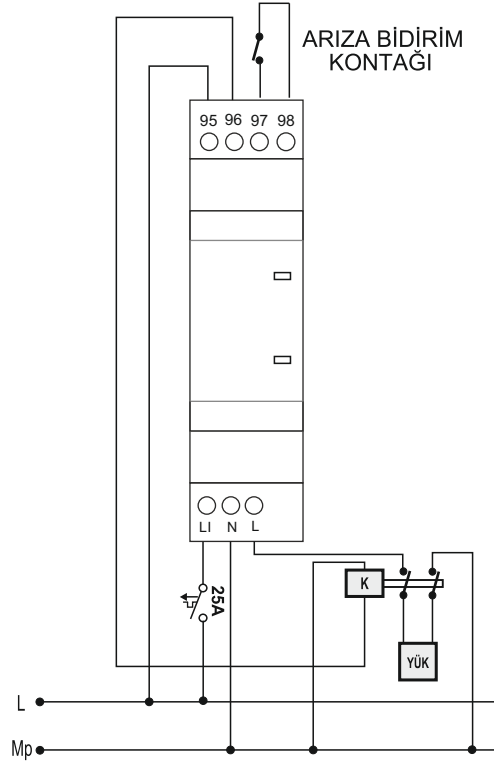
Şekil 2: Bağlantı Şeması
